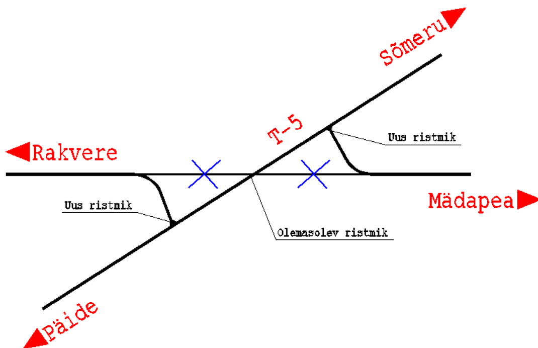
Joonis 6. Maantee nr 17149 Rakvere– Jõepere ja nr 5 Pärnu-Rakvere-Sõmeru ristmiku rekonstrueerimise põhimõtteline eskiislahendus. OÜ Reaalprojekt, aprill 2009
